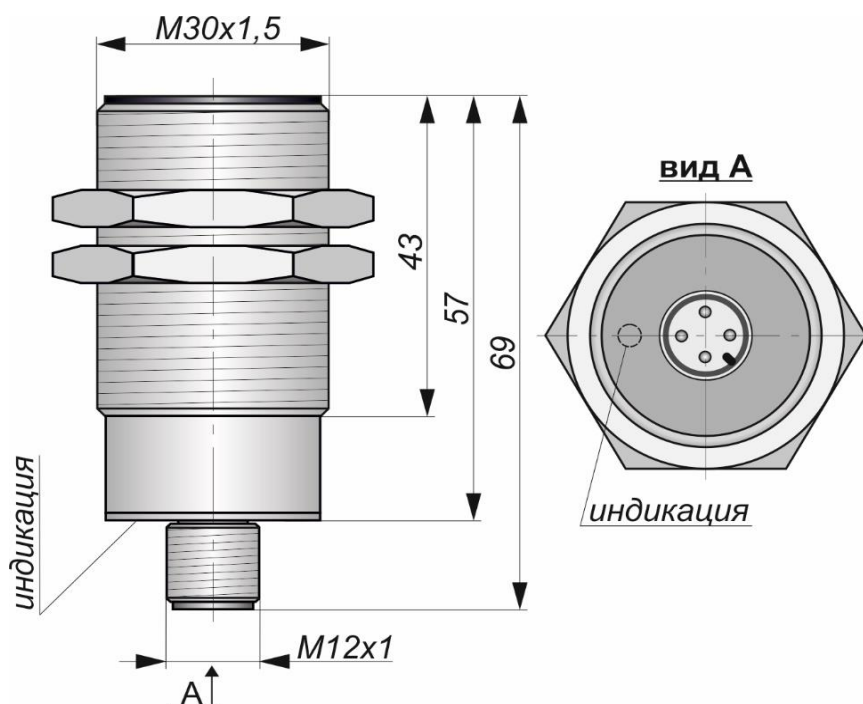
Габаритный чертеж
